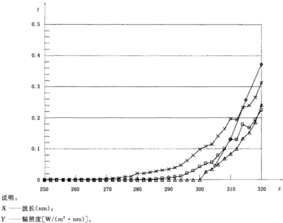
图 2 使用 1 型(□)、2 型(△)、3 型(×)滤光器的开放式碳弧灯与 CIE 85:1989 表 4 中的日光(◇)从 250 nm~320 nm 的典型光谱辐照度比较
